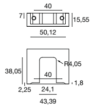
Foratura ripiano / Shelf machining
