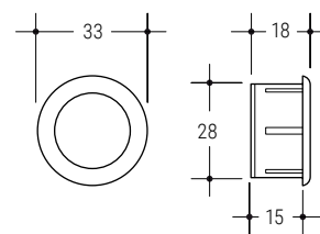
362 Senza fondo Without base Ø 33 h 15 VE VS VG VM SP
