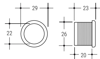
087 Senza fondo Without base Ø 29 h 20 VE VS VG GA SP
