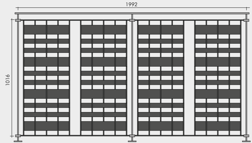
railing applications applicazione per parapetti
