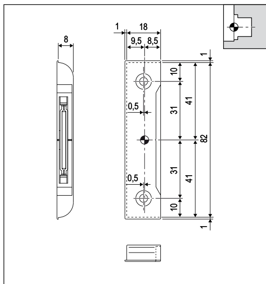
Parte telaio, aria 4 mm, interasse 9 mm
