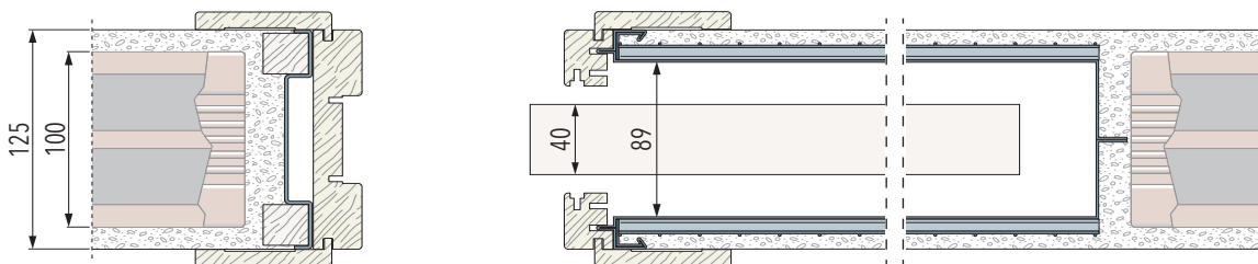
Parete Finita 125 mm - Tramezza 100 mm
