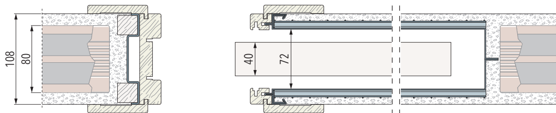
Parete Finita 108 mm - Tramezza 80 mm
