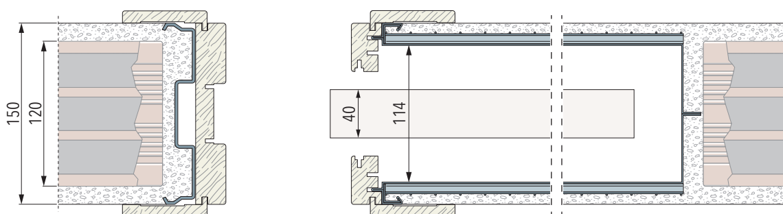
Parete Finita 150 mm - Tramezza 120 mm
